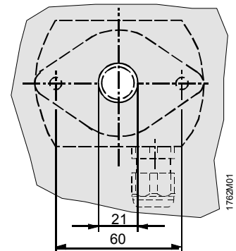
Otwory montażowe
