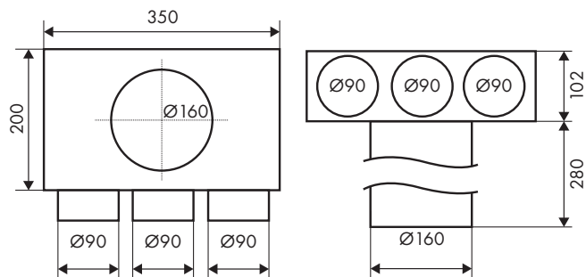
FLEXO BOX PRO T3 — 3×Ø90/Ø160
