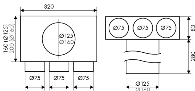
FLEXO BOX PRO T3 – 3×Ø75 / Ø125–160
