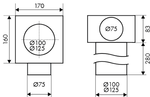
FLEXO BOX PRO T1 – 1×Ø75 / Ø100–125
