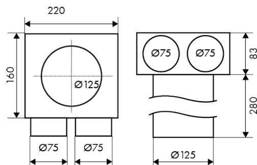
FLEXO BOX PRO T2 – 2×Ø75 / Ø125
