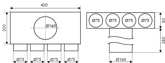
FLEXO BOX PRO T4 – 4×Ø75 / Ø160
