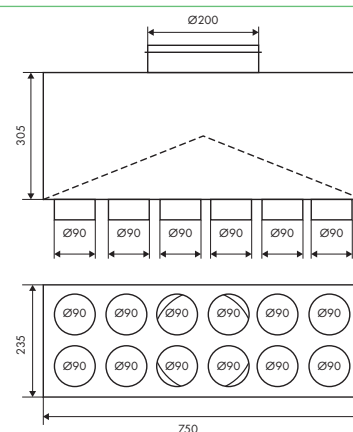
FLEXO BOX PRO P12x90/200
