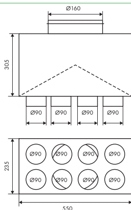
FLEXO BOX PRO P8x90/160
