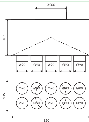
FLEXO BOX PRO P10x90/200
