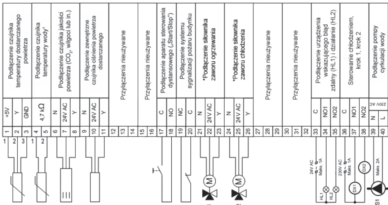
Schemat podłączenia elementów zewnętrznych systemu sterowania
