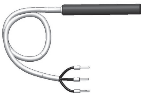
Czujnik temperatury powietrza nawiewanego B1
