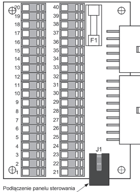
Schemat podłączenia elementów zewnętrznych systemu sterowania
