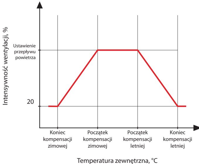
Rysunek 1. Działanie funkcji OCV
