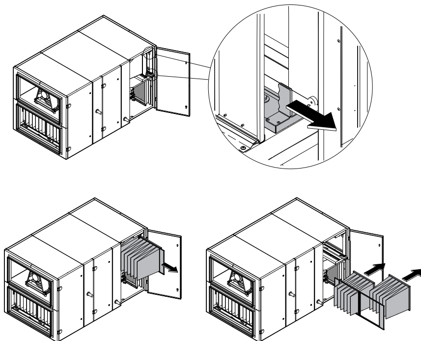
Rysunek 3. Urządzenie mocujące filtr
