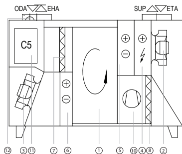
Prawa strona inspekcyjna R1
