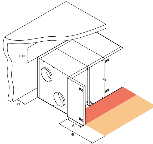
Rys. 8. Obszar inspekcji urządzenia
