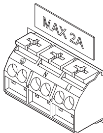
Rys. 25. Dodatkowy blok złącz
