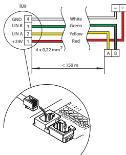
Rys. 19. Schemat okablowania panelu sterowniczego
