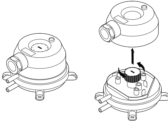
Rys. 24. Przełącznik ciśnieniowy
