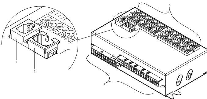
Rys. 14. Płyta główna sterownika C5
