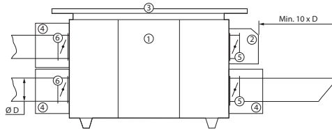
Rys.13 Akcesoria do central wentylacyjnych montowanych na zewnątrz
