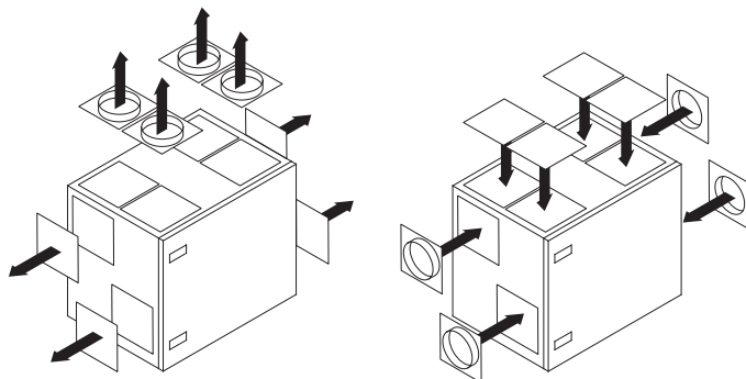
Rys. 5. Przeniesienie króćców przyłączeniowych kanałów central uniwersalnych
