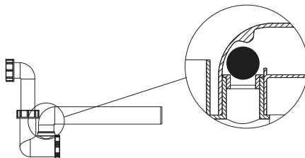
Rys. 11. Przykład syfonu z zaworem jednokierunkowym
