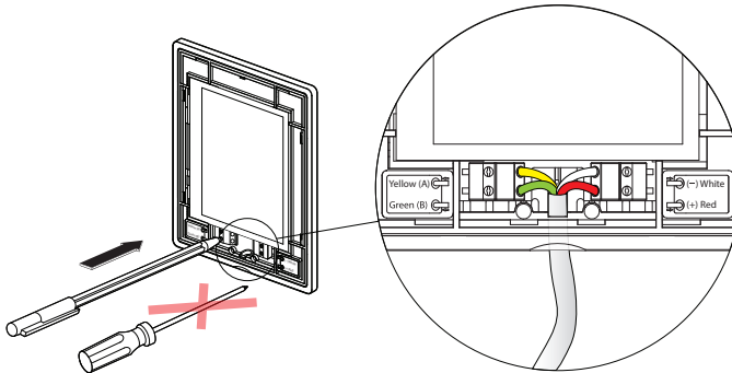
Rys. 20. Schemat okablowania panelu sterowniczego
