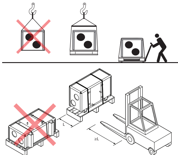
Rys. 7. Przykłady transportu dźwigiem, wózkiem widłowym lub paletowym
