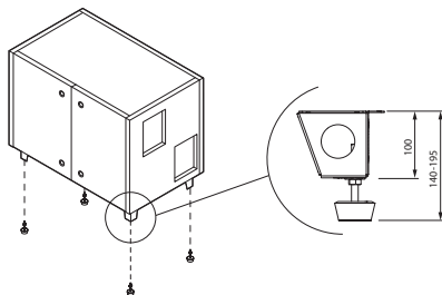
Rys. 7. Jednostka wentylacyjna z nogami montażowymi i regulowanymi stopkami
