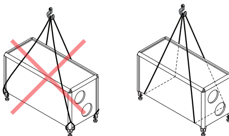
Rys. 6. Transport dźwigiem
