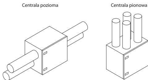
Rys. 4. Klasyfikacja central według podłączenia kanałów
