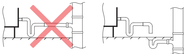
Rys. 12. Przyłącze spustu kondensatu do instalacji kanalizacyjnej
