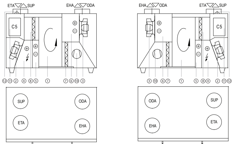
Lewa strona inspekcyjna L1
