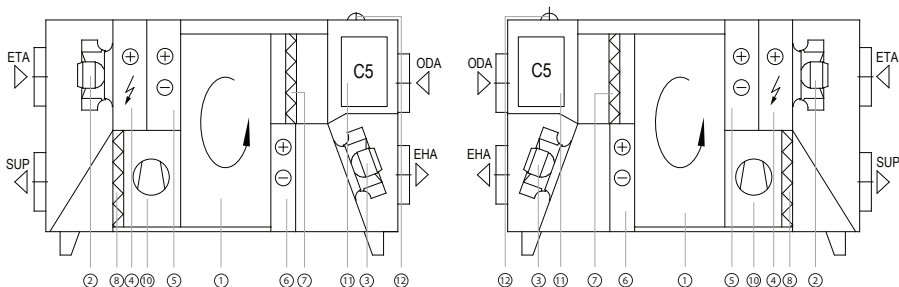
Lewa strona inspekcyjna L1
