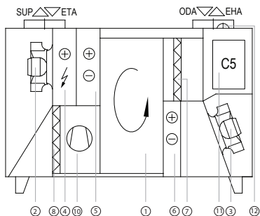
Lewa strona inspekcyjna L1
