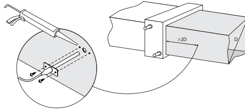
Rys. 18. Montaż czujnika temperatury powietrza nawiewanego
