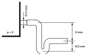
Rys. 10. Montaż syfonu
