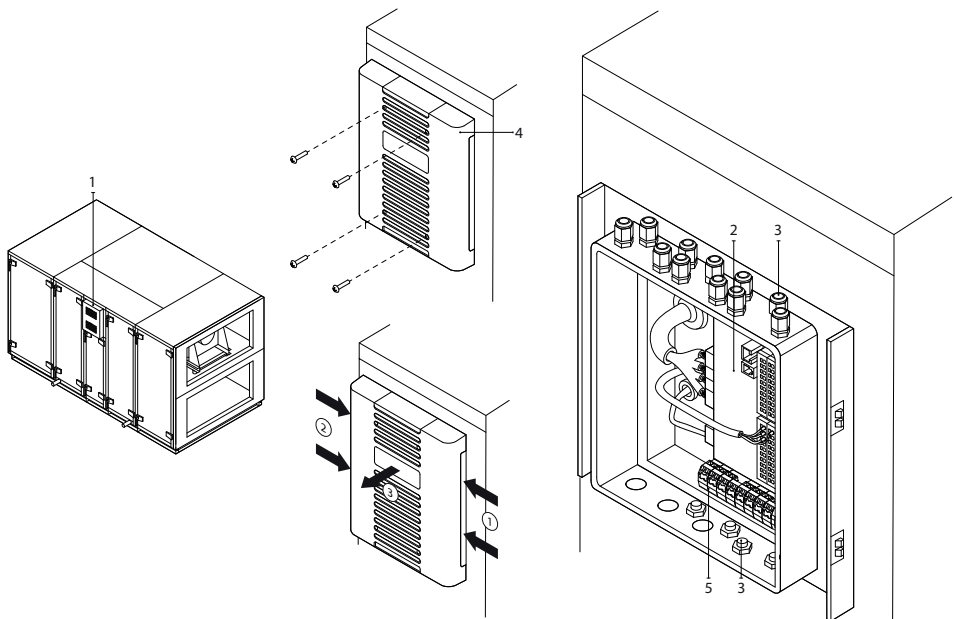
Rys. 37. Skrzynka automatyki
