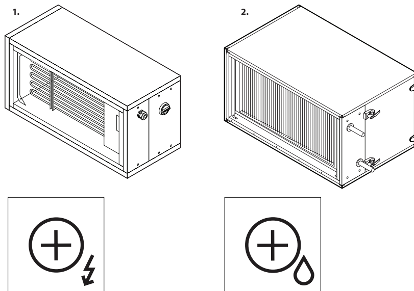
Rys. 8. Sekcja nagrzewnicy
