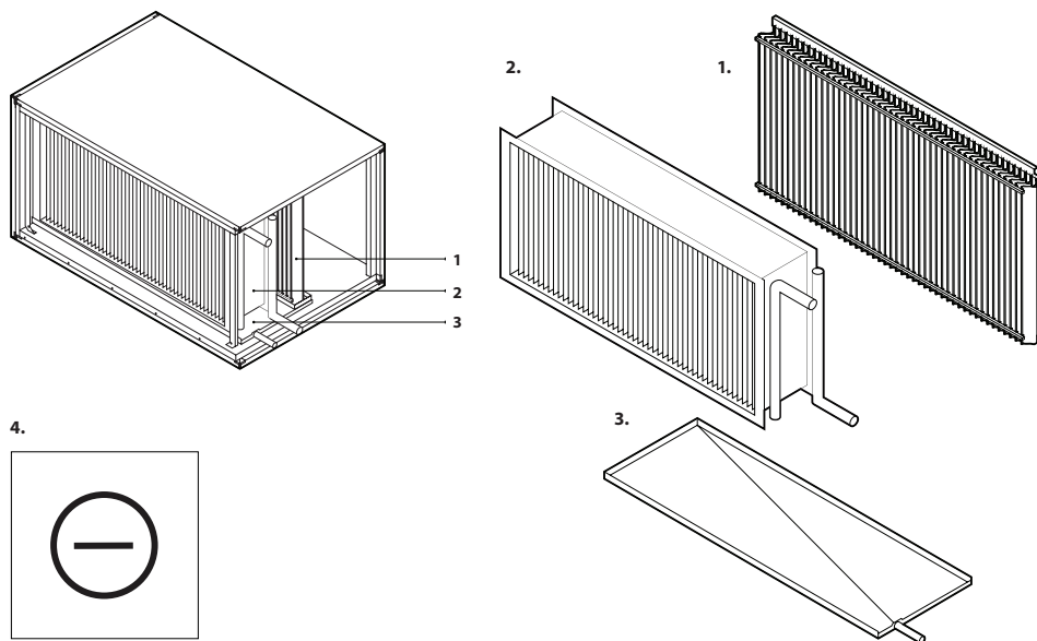
Rys. 7. Sekcja chłodnicy
