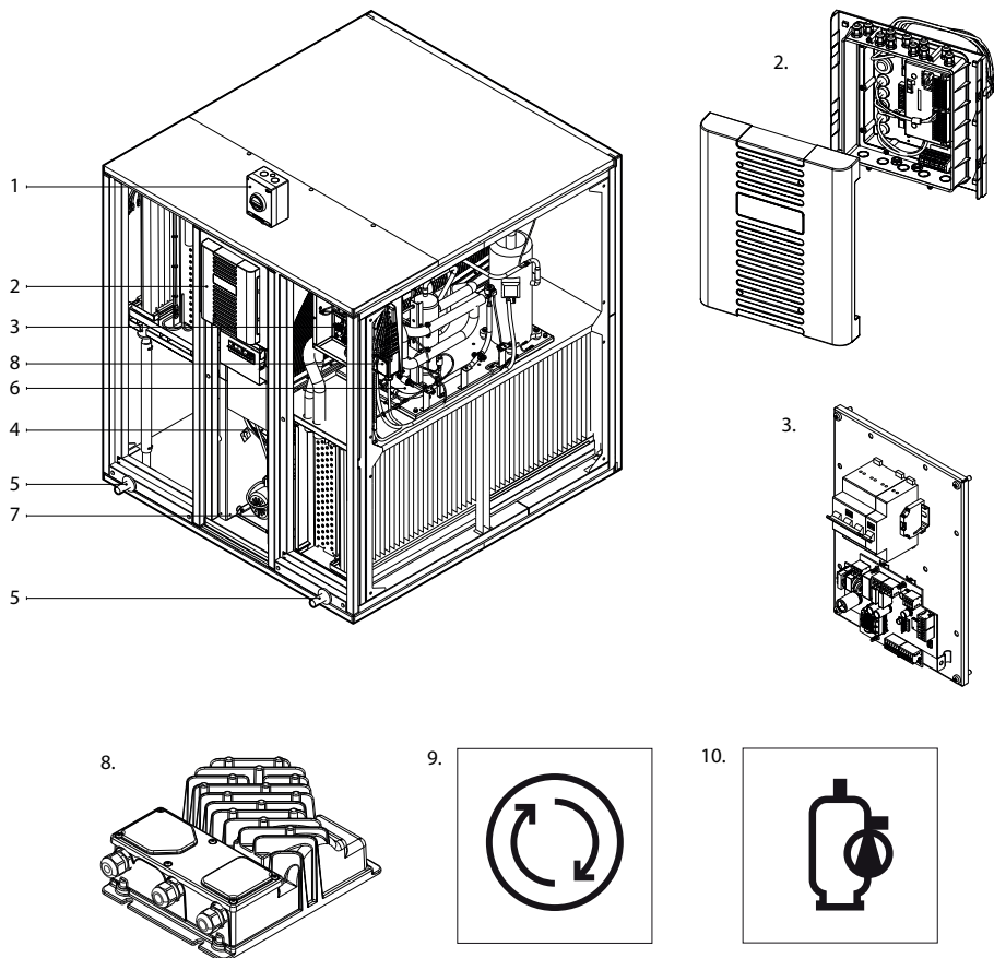
Rys. 2. Sekcja pompy ciepła
