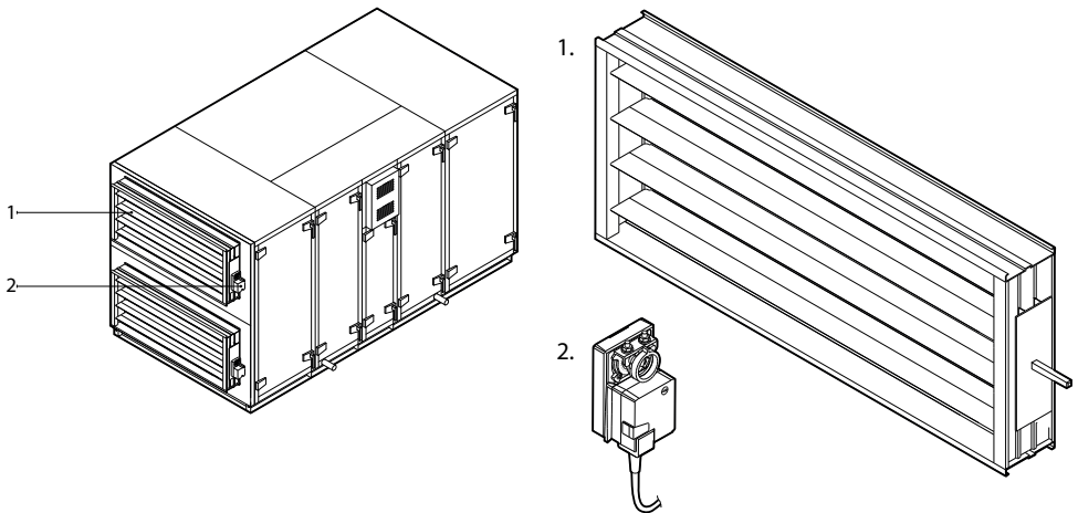
Rys. 9. Przepustnica zamykająca przepływ powietrza 1 – przepustnica powietrza, 2 – elektryczny siłownik przepustnicy
