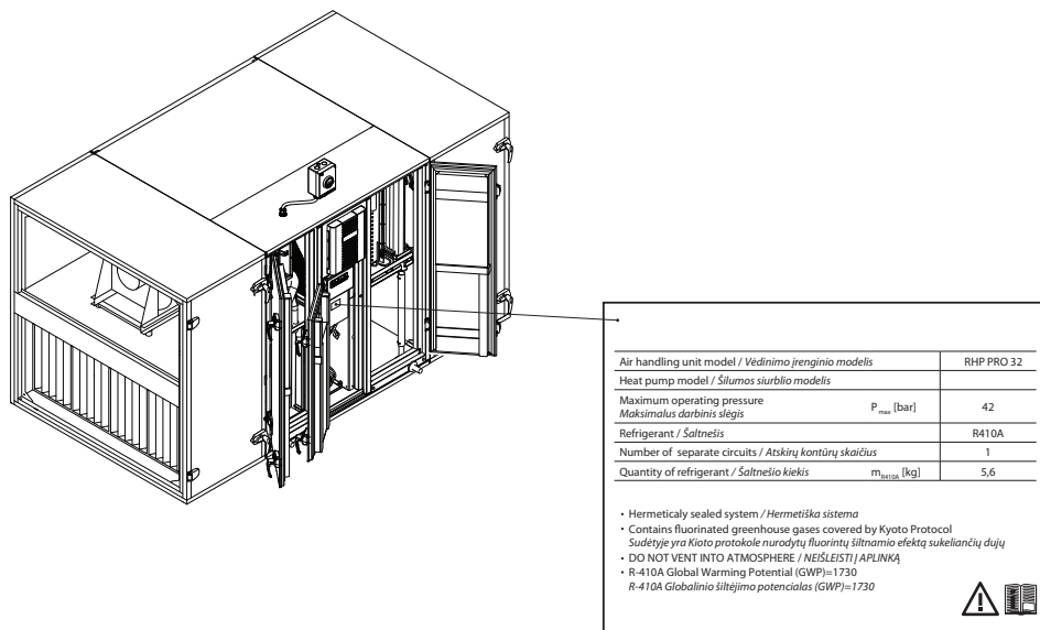
Rys. 5. Przykład tabliczki informacyjnej pompy ciepła
