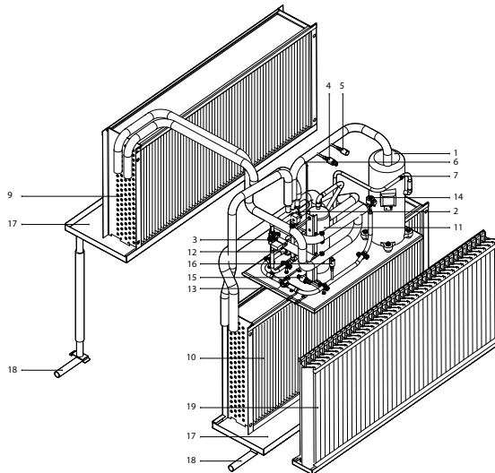
Rys. 4. Schemat obrotu hydraulicznego i podzespołów pompy ciepła
