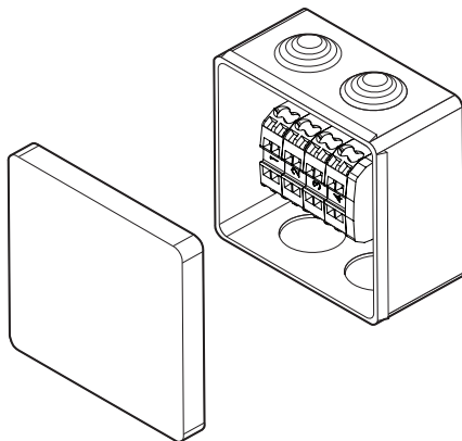
Rys. 49. Skrzynka przyłączeniowa PD1
