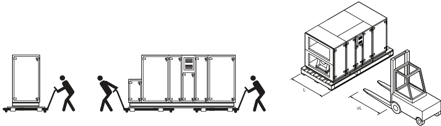
Rys. 13. Transport centrali wózkiem widłowym lub paletowym
