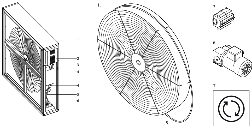
Rys. 3. Sekcja rekuperatora obrotowego
