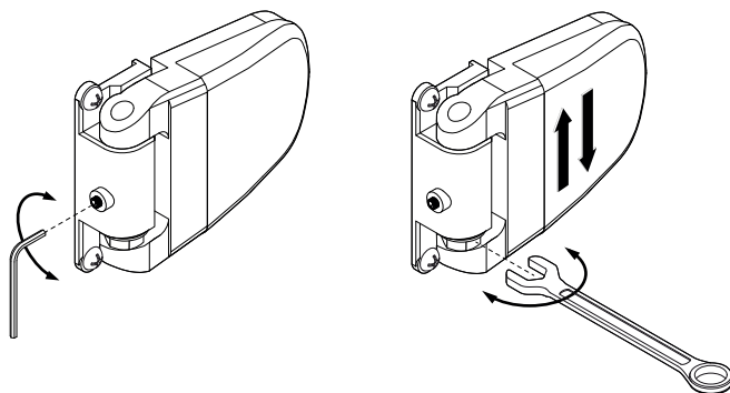
Rys. 20. Regulacja zawiasów
