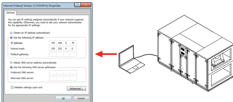
Rys. 51. Ustawienia sieci komputerowej do bezpośredniego połączenia z centralą
