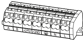
Rys. 44. Dodatkowa listwa zaciskowa
