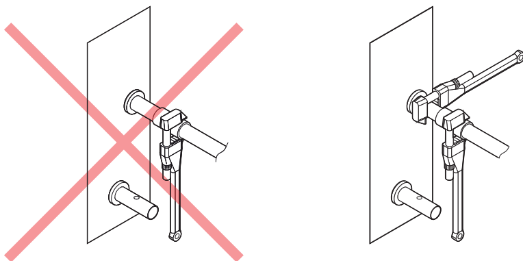
Rys. 25. Podłączanie tulei
