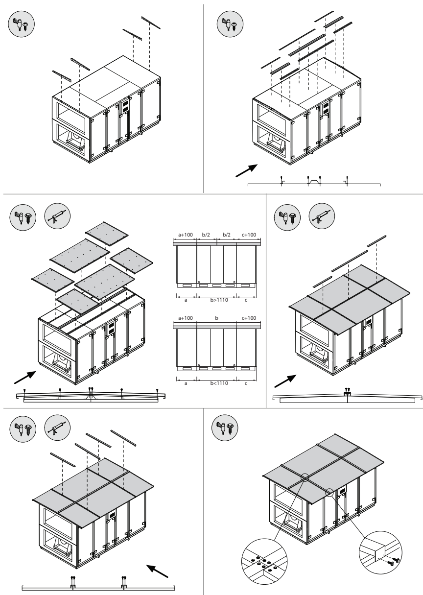
Rys. 34. Montaż osobno zamawianego dachu ochronnego 1
