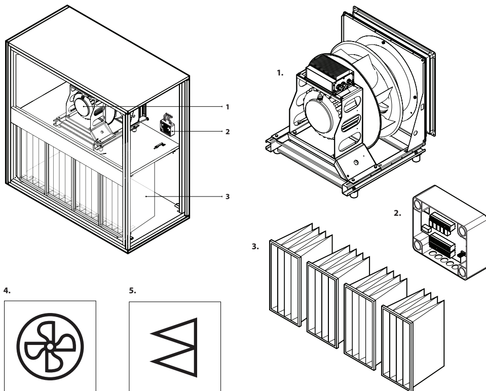
Rys. 1. Sekcja filtr-wentylator
