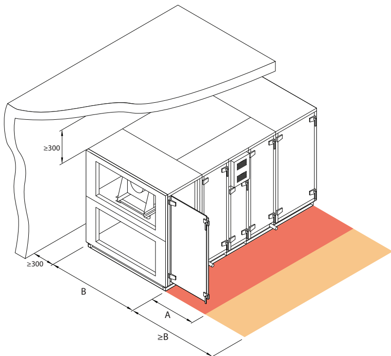
Rys. 18. Obszar inspekcji urządzenia
