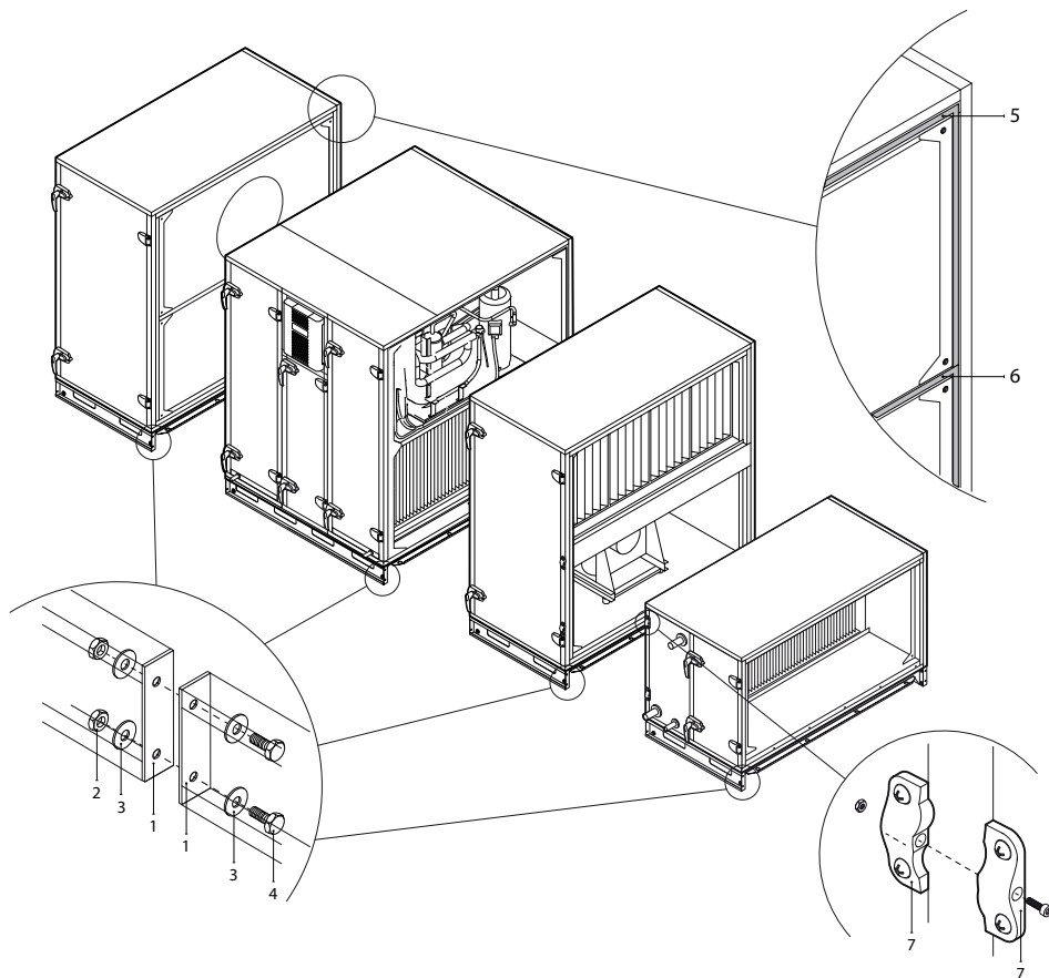
Rys. 21. Zewnętrzne połączenie i uszczelnienie sekcji
