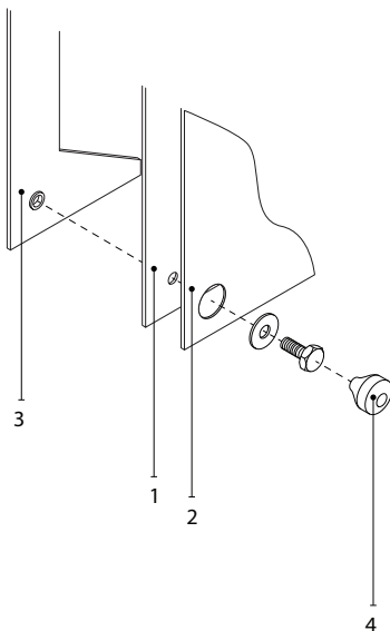
Rys. 23. Połączenie wewnętrzne w sekcji wentylatora
