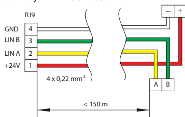
Rys. 46. Schemat okablowania panelu sterowniczego
