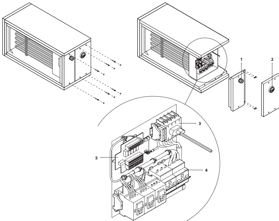
Rys. 36. Wyłącznik główny wewnątrz sekcji nagrzewnicy elektrycznej
