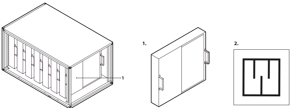
Rys. 10. Sekcja tłumienia hałasu 1 – zdejmowane przegrody pochłaniające hałas, 2 – oznaczenie sekcji tłumika
