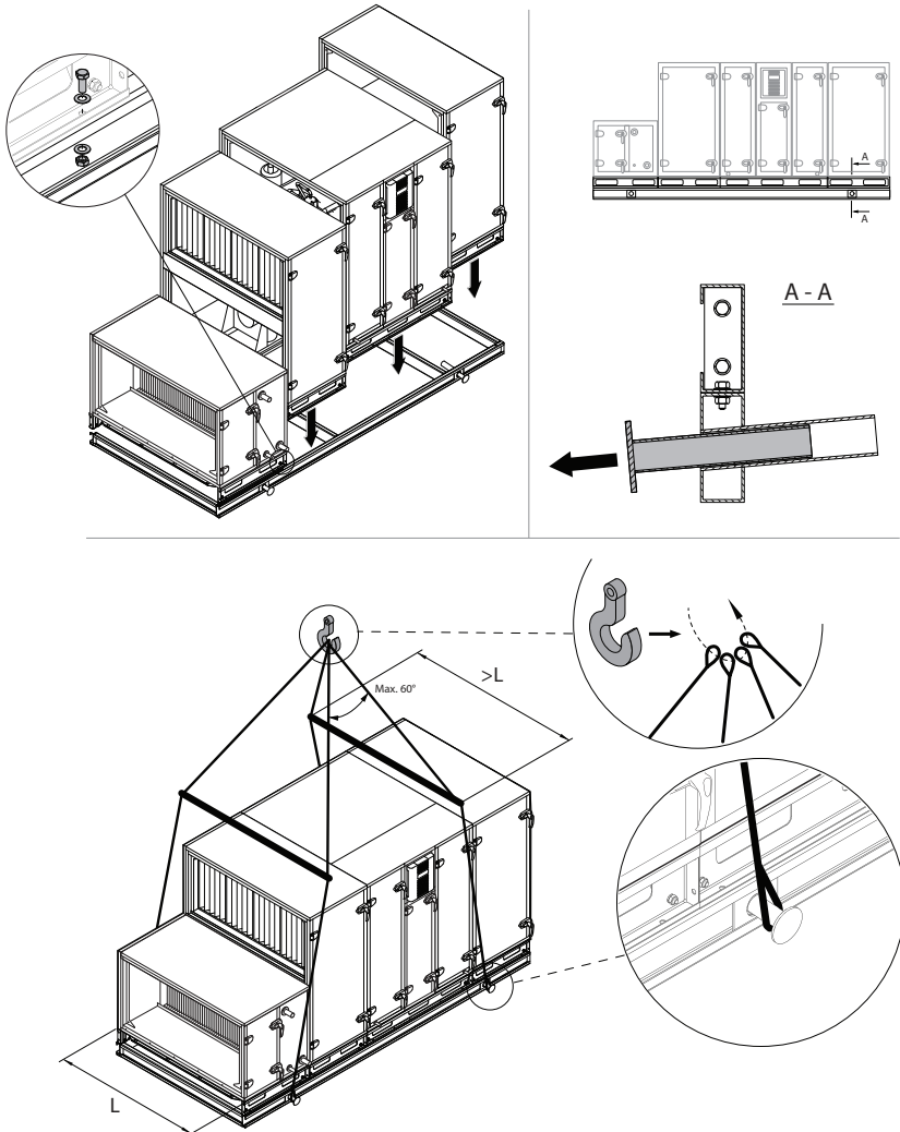
Rys. 15. Podnoszenie w pełni zmontowanej centrali na wzmocnionej ramie montażowej 1
