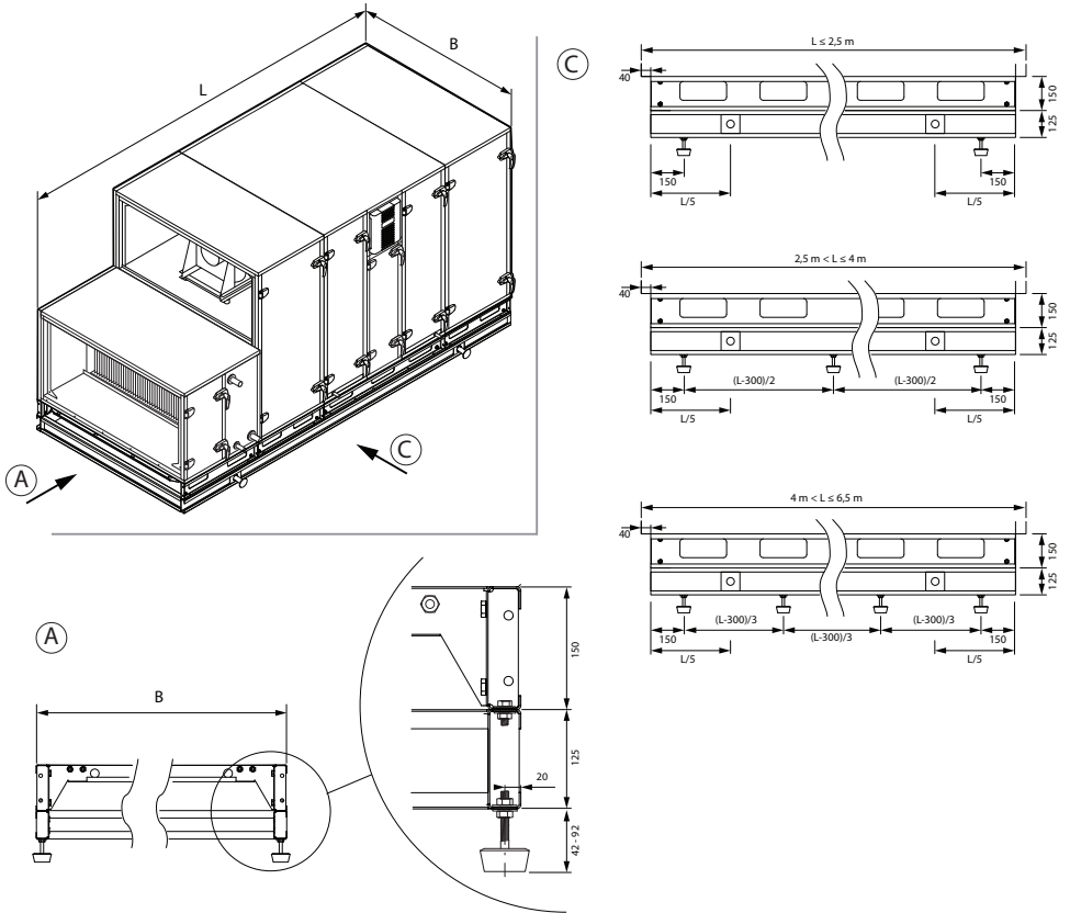
Rys. 16. Wymiary wzmocnionej ramy montażowej
