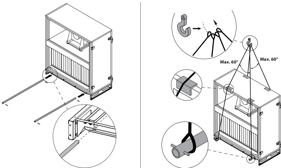
Rys. 14. Podnoszenie poszczególnych sekcji 1
