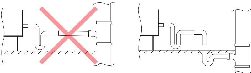
Rys. 30. Przyłącze spustu kondensatu do instalacji kanalizacyjnej
