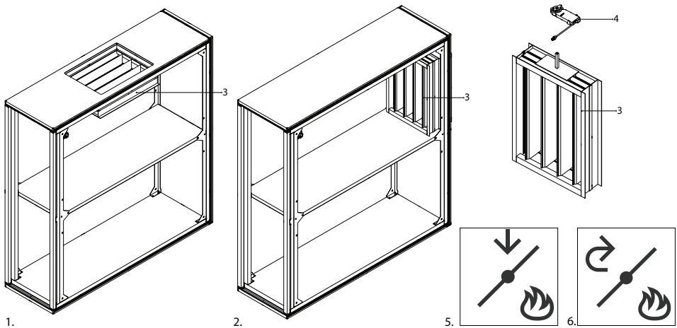
Rys. 12. Sekcja oddymiania
