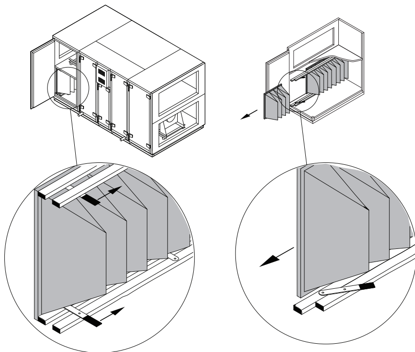
Rys. 53. Urządzenie mocujące filtr
