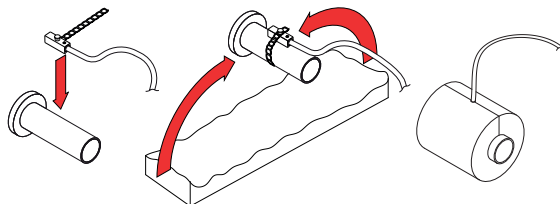
Rys. 26. Montaż nawierzchniowego czujnika temperatury wody powrotnej 2
