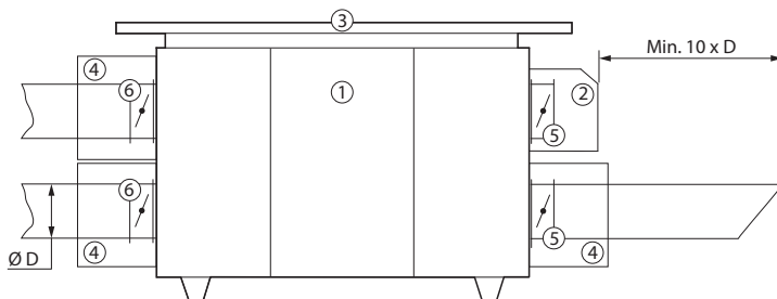
Rys. 33. Akcesoria do central wentylacyjnych montowanych na zewnątrz
