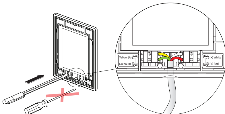
Rys. 47. Schemat okablowania panelu sterowniczego
