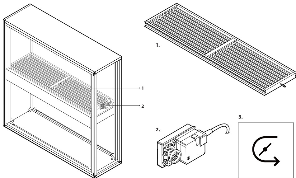
Rys. 6. Sekcja recyrkulacji
