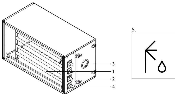
Rys. 11. Sekcja nawilżacza
