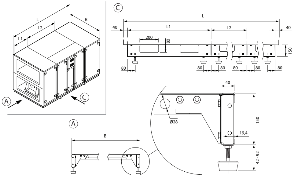
Rys. 17. Rama montażowa z regulowanymi nóżkami
