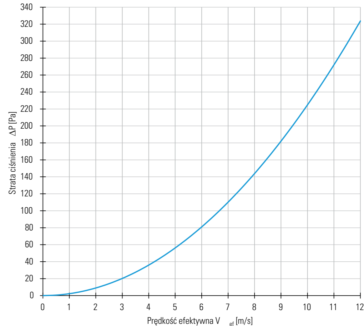
Strata ciśnienia \Delta P [Pa]
