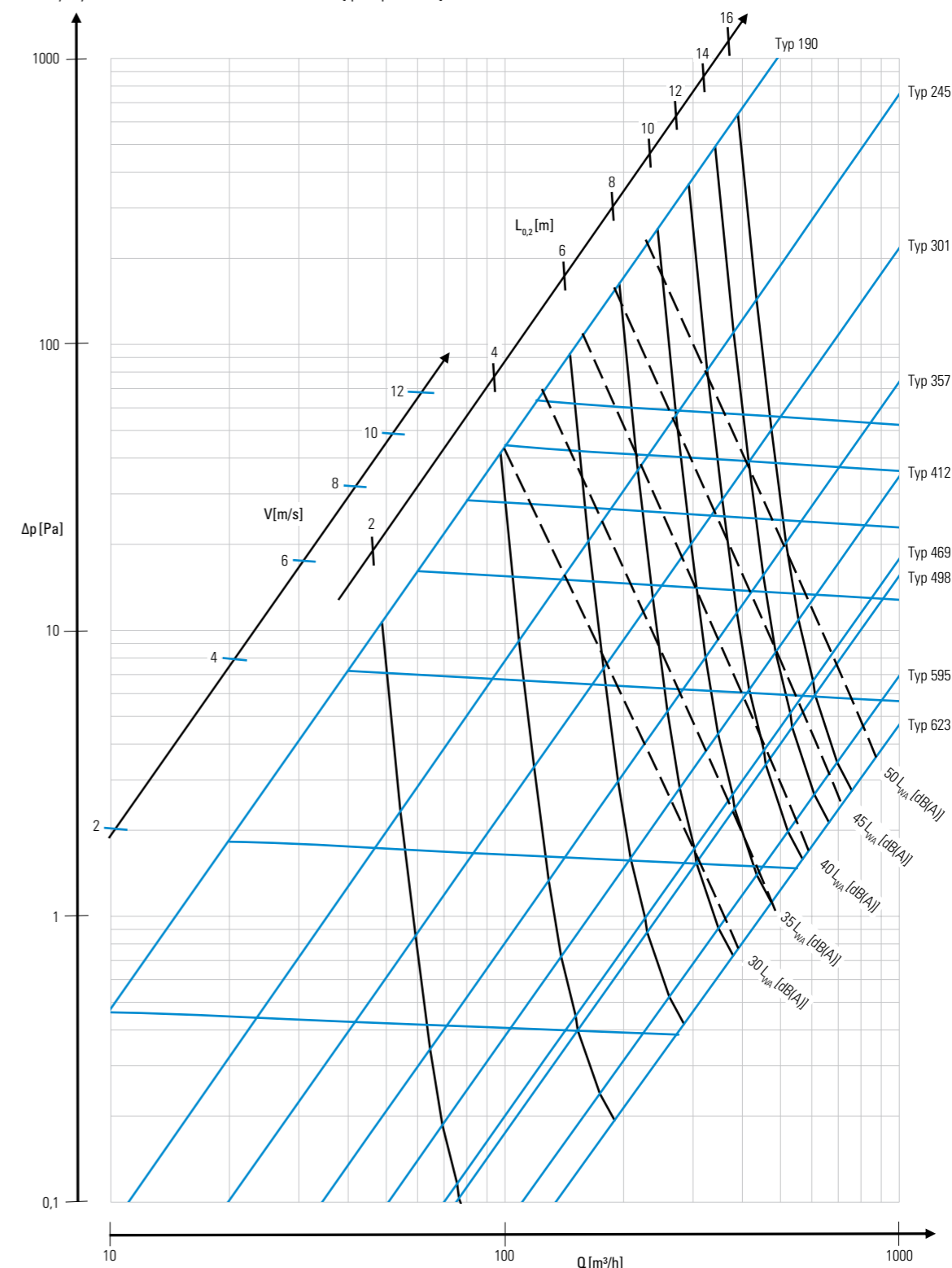
L - Zasięg strumienia o max. V=0,25 \text{ m/s} . Średnia V strumienia 0,08-0,10 \text{ m/s} .
