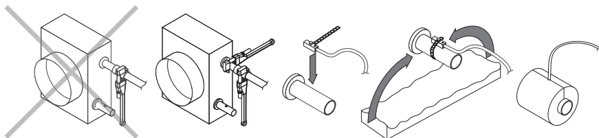
Rys. 16. Podłączanie przewodów nagrzewnicy/chłodziwy wodnej i instalowanie czujnika temperatury wody powrotnej
